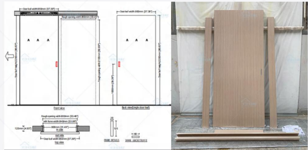
Barn door
