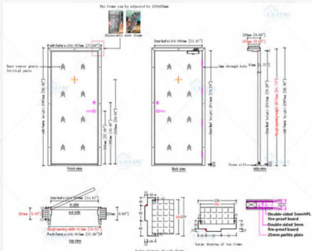
UL 20 min Wooden Fire Door
