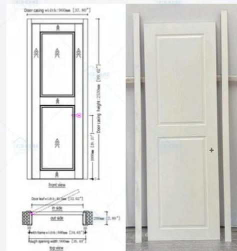
Bedroom Door
