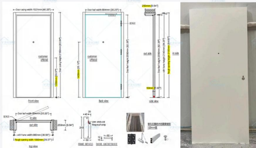
UL FD45 min Hotel Room Door
