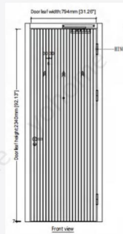
UL 45 min Wooden Fire Door
