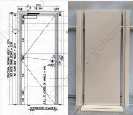
UL 45 min Wooden Fire Door
